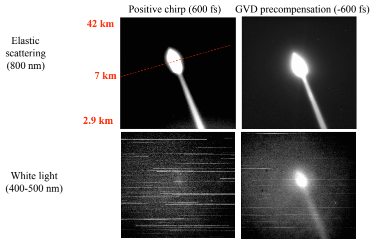
Figure. 1. Images du faisceau laser dans deux gammes de longueurs d'onde (fondamentale et continuum de lumière blanche), pour deux impulsions de même durée mais de chirps opposés
